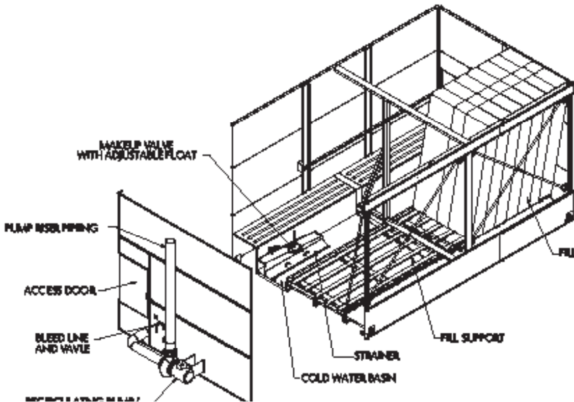
BOTTOM-PAN SECTION
